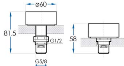
SPIN/MESH In Wall Top Assemblies Set SP161-CH / SP161-MB / SP161-BB / SP161-BN SPM161-CH / SPM161-MB / SPM161-BB / SPM161-BN
